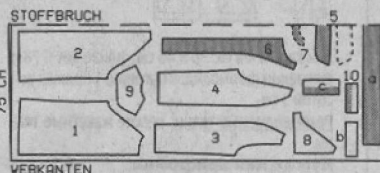
План раскладки при ширине ткани 150 см
