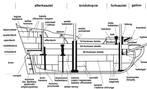
przekrój kadłuba galeonu z XVIII w.
