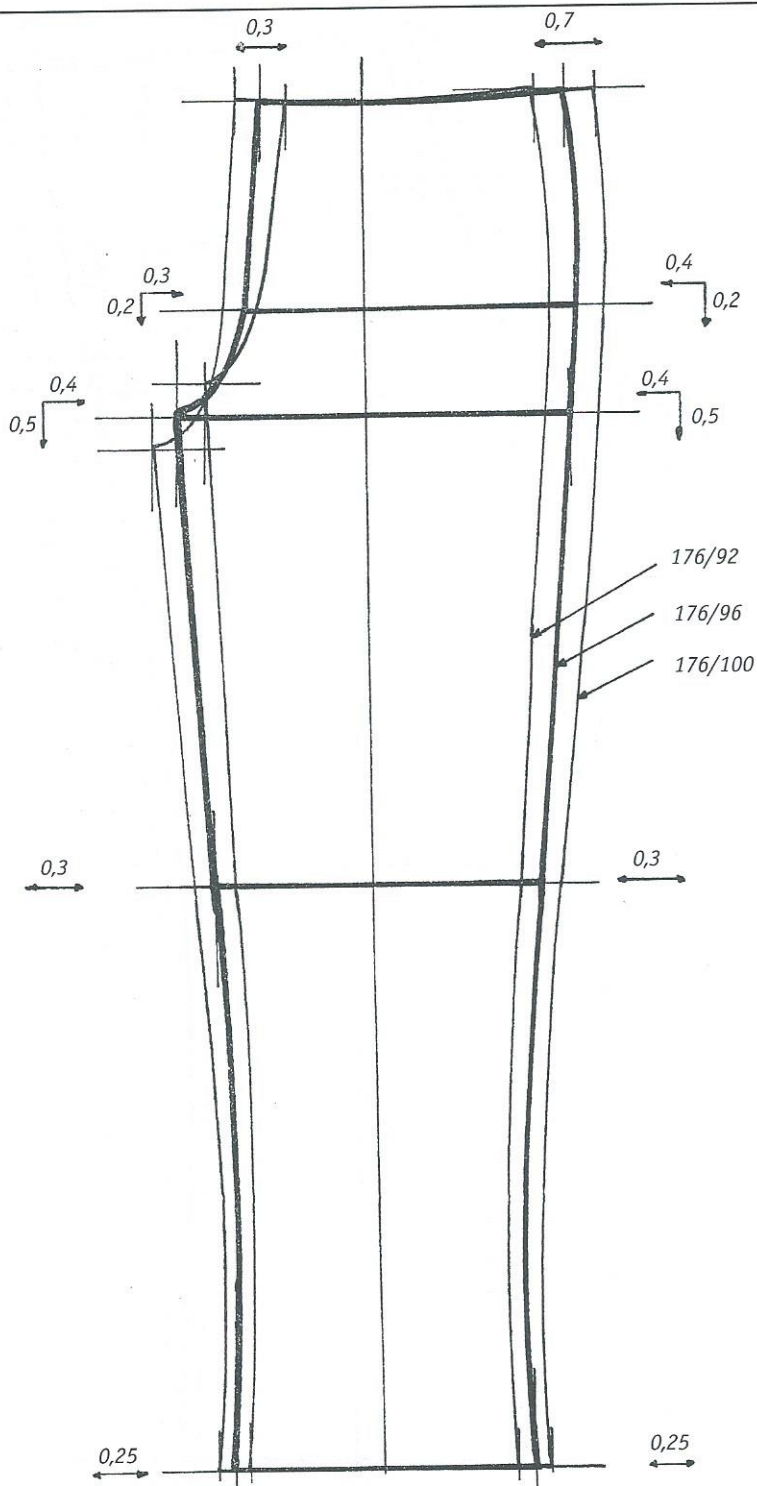
Rys. 92. Stopniowanie obwodowe przedniej nogawki spodni.
