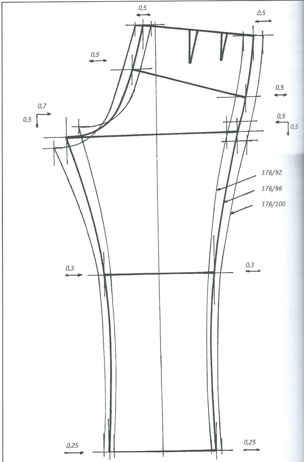
Rys. 93. Stopniowanie obwodowe tylnej nogawki spodni.
